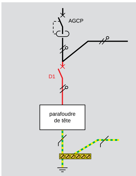
b. le parafoudre se déconnecte en cas de court circuit
