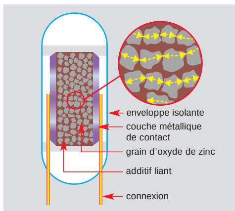
varistance à oxyde de zinc
