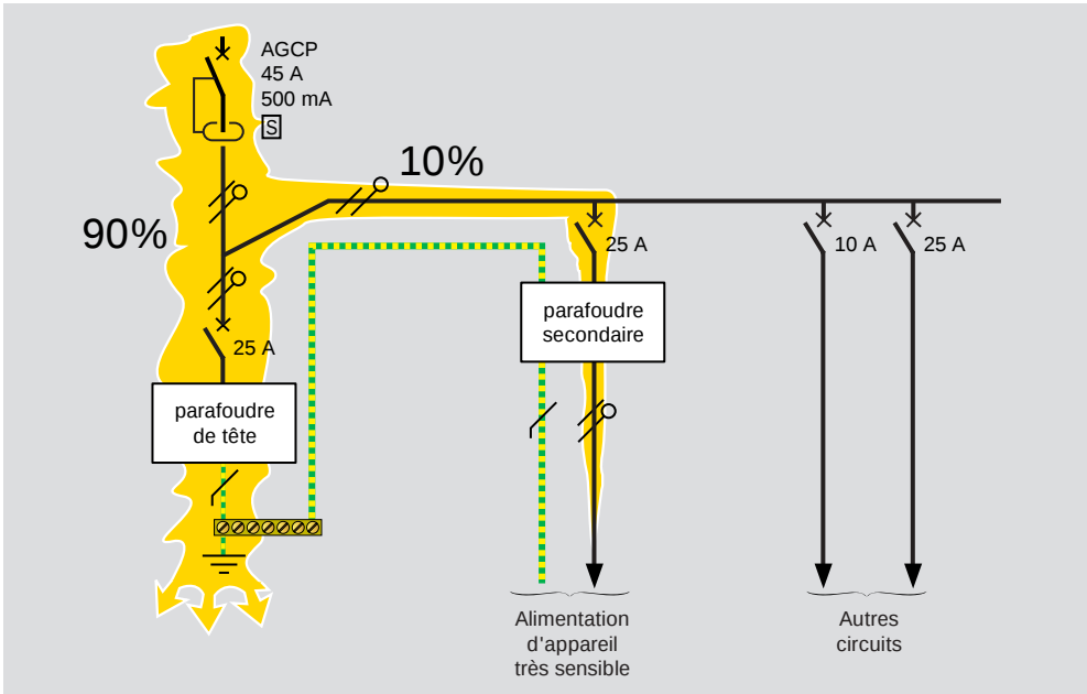
schéma de principe : protection de tête et protection fine
