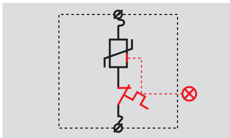
a. le parafoudre se déconnecte en cas d'emballement thermique
