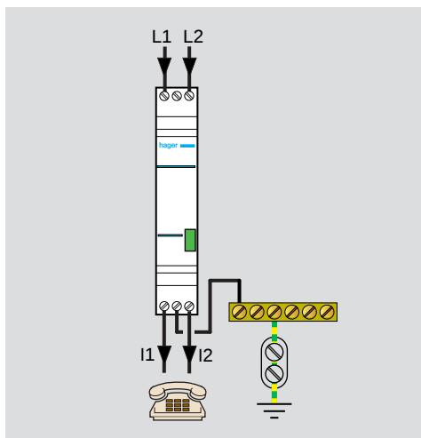
mise en œuvre d'une protection téléphonique
