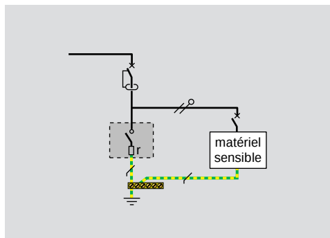
schéma 1 : fonctionnement normal
