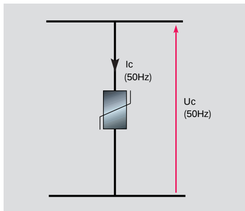
schéma 1 : caractéristiques aux bornes d'une branche du parafoudre en fonctionnement normal (50Hz, 230/400V)
