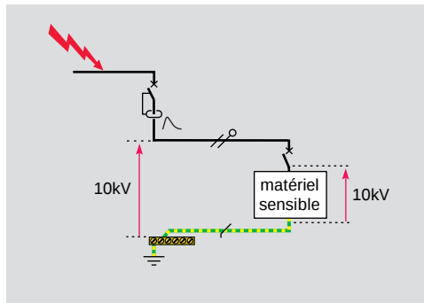
schéma 1 : sans parafoudre, la surtension apparaît aux bornes des matériels
