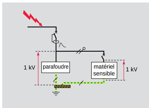
schéma 4 : le parafoudre limite la surtension aux bornes du matériel
