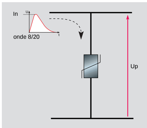
schéma 2 : caractéristiques aux bornes d'une branche du parafoudre pendant l'écoulement de la surtension
