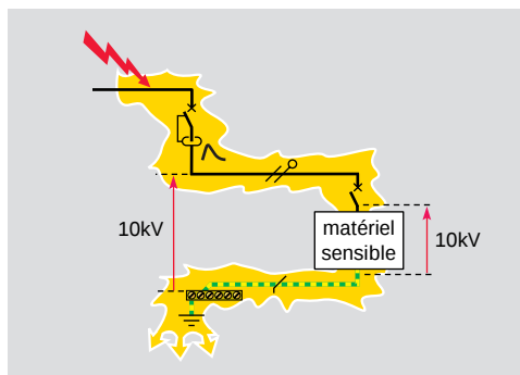
schéma 2 : sans parafoudre, le matériel "claque"
