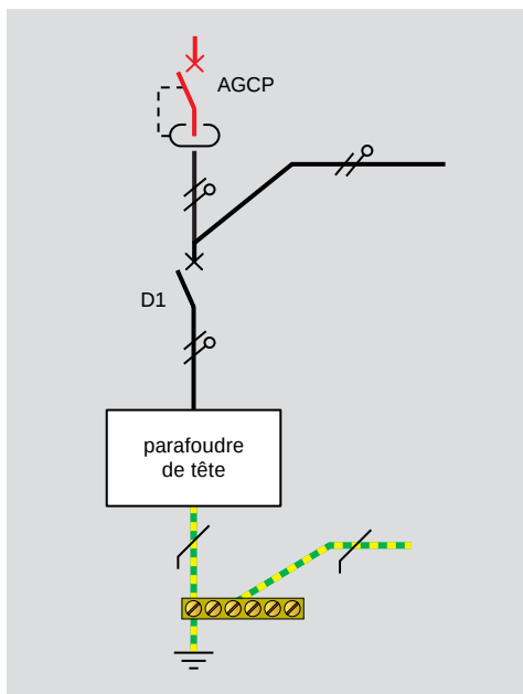
parafoudre de tête directement en aval de l'AGCP
