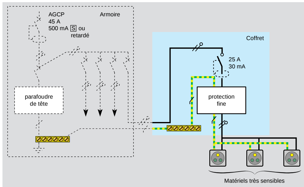
utilisation d'un coffret divisionnaire proche du matériel à protéger
