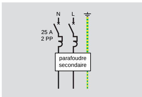
protection bipolaire d'un parafoudre secondaire
