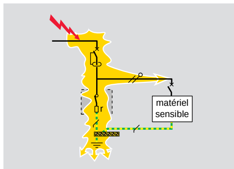
schéma 2 : pendant la surtension
