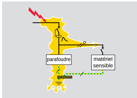
schéma 3 : écoulement de "l'énergie foudre" à la terre
