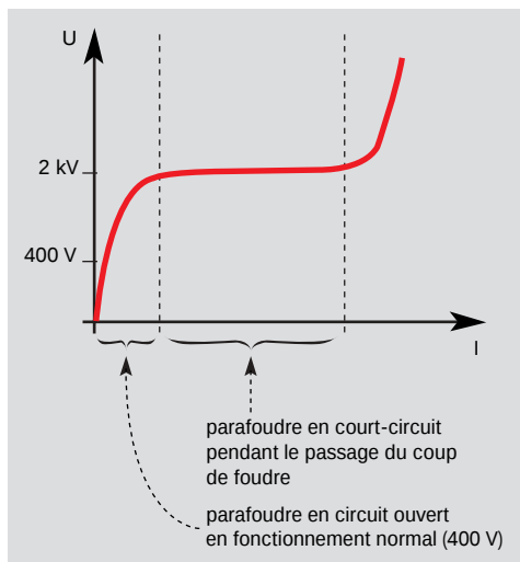
tension aux bornes d'une varistance en fonction de l'intensité "écoulée"
